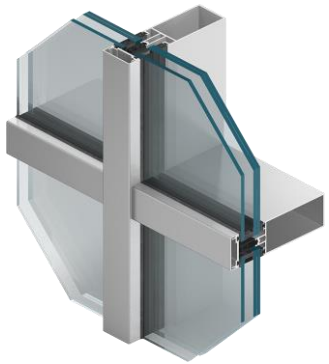
MB-SR50N A függönyfalak
