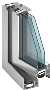
MB-86 SI ablakok
