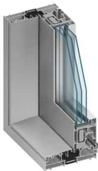
MB-77 HS emelő-toló ajtók
